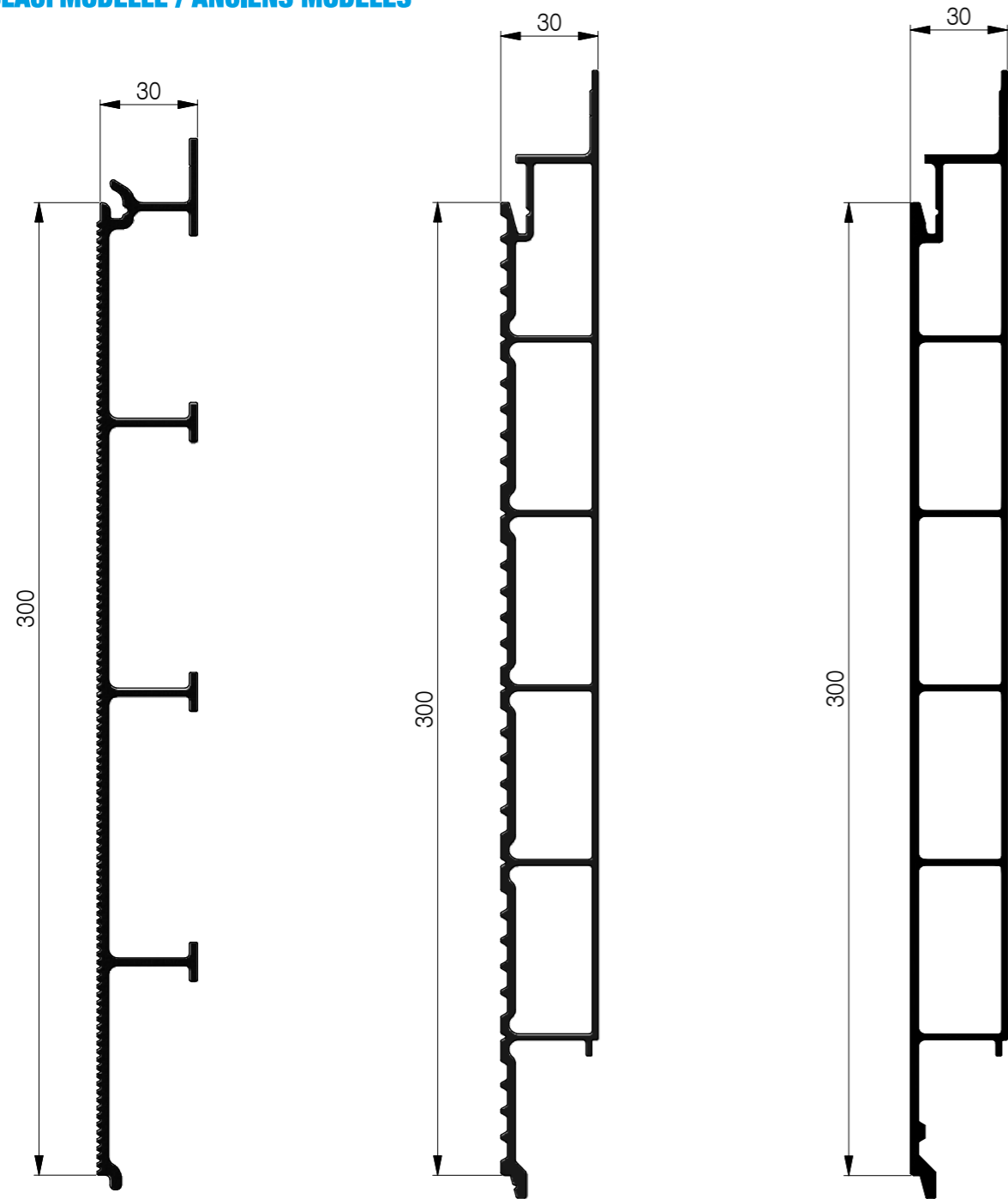
51 024 3.965 kg/m L = 6350 R
