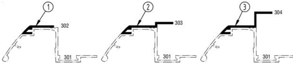
Dachabdeckprofil
