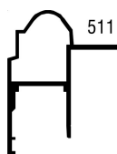
Dachanschlussprofil
