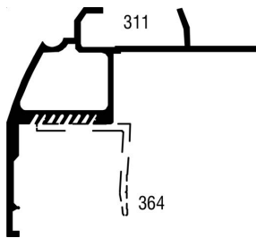
Dachanschlussprofil
