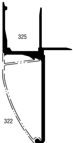
Bodenrahmenprofil
