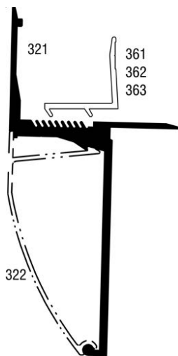
Bodenrahmenprofil
